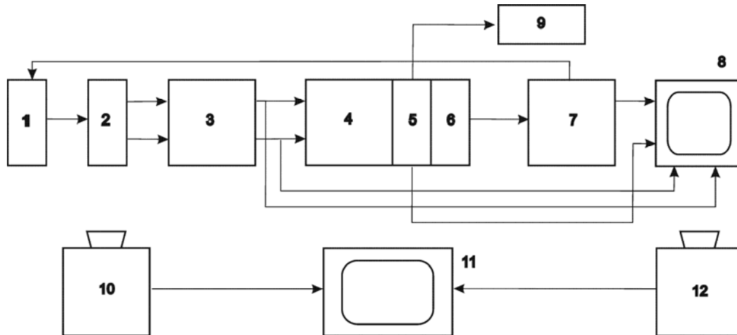
Рис. 1. Структурна схема комплексу для електростимуляції під час виконання легкоатлетичних стрибків:
