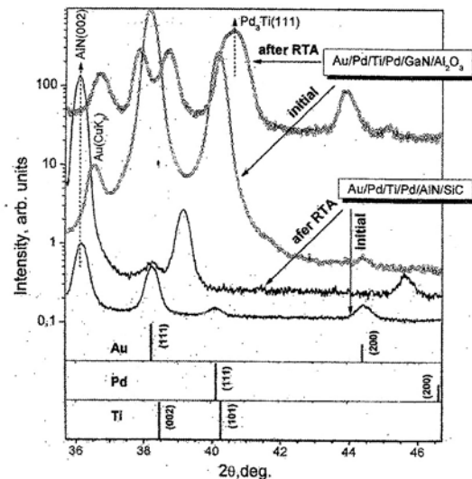
Рис. 2. Рентгенодифрактограма омичних контактів Au-Pd-Ti-Pd/AlN/SiC та Au-Pd-Ti-Pd/GaN/ \text{Al}_2\text{O}_3
