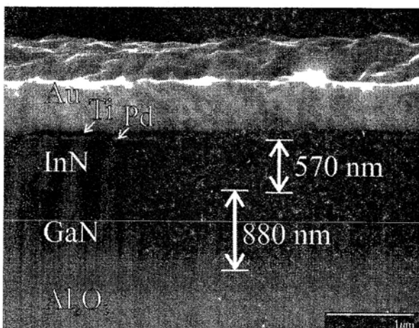
Рис. 1. Скол контактної структури Au-Pt-Ti-n-InN/GaN/ \text{Al}_2\text{O}_3
