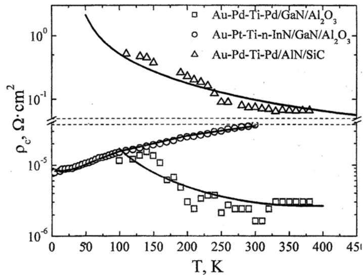
Рис. 3. Залежність питомого контактного опору від температури омичних контактів до к n-AlN, n-GaN, n-InN
