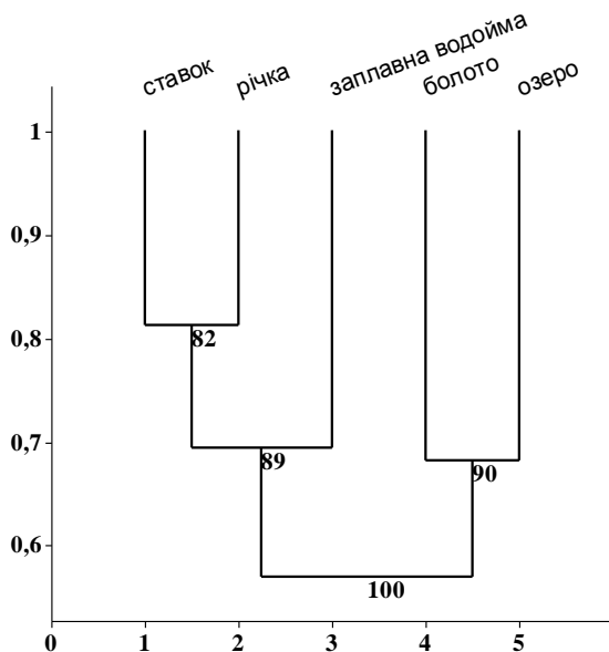
Рис. 1. Дендрограма подібності видового складу черепашкових амеб різних типів водойм за індексом Чекановського-С'єренсена. Цифри у вузлах дендрограми – вірогідність у відсотках даних кластерів за результатами Bootstrap-аналізу при 1000 перестановок.
