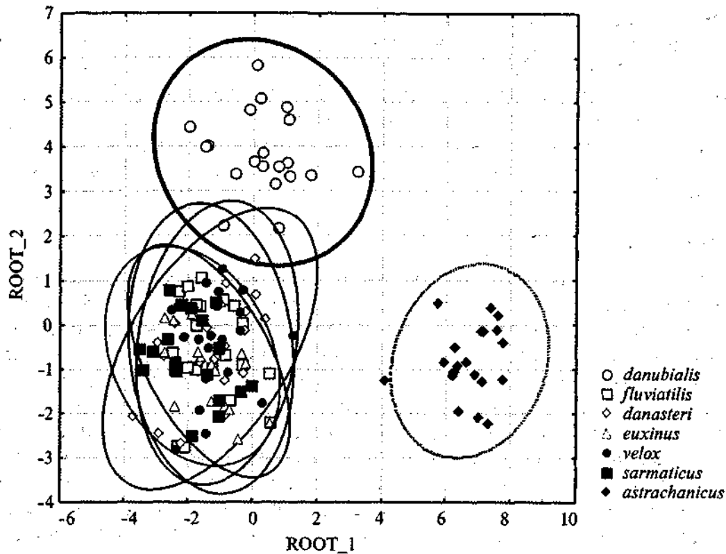
Рис. 2. Изменчивость семи предполагаемых видов рода Theodoxus по комплексу признаков раковины, крышечки и органов половой системы в пространстве первых двух канонических переменных (ROOT_1, ROOT_2).
