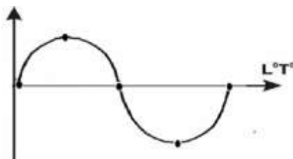
Рис. Синусоидальная модель реальности в общем виде
