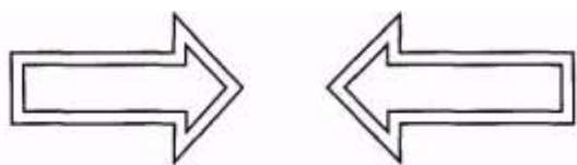
Рис. Точечный Аттрактор
