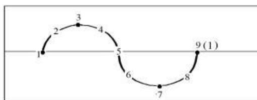
Рис. 8. Структура волны
