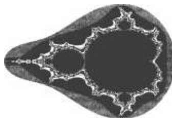
Рис. Странный Аттрактор
