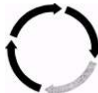
Рис. Циклический (Круговой) аттрактор.
