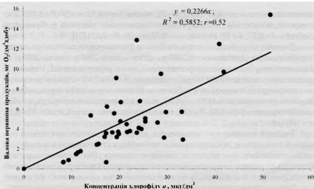
Рис. 2. Залежність між вмістом хлорофілу a та валовою первинною продукцією фітопланктону р. Тетерів (за даними досліджень 2005—2006 рр., n = 49 ). Розрахунок проведено для горизонту максимального фотосинтезу
