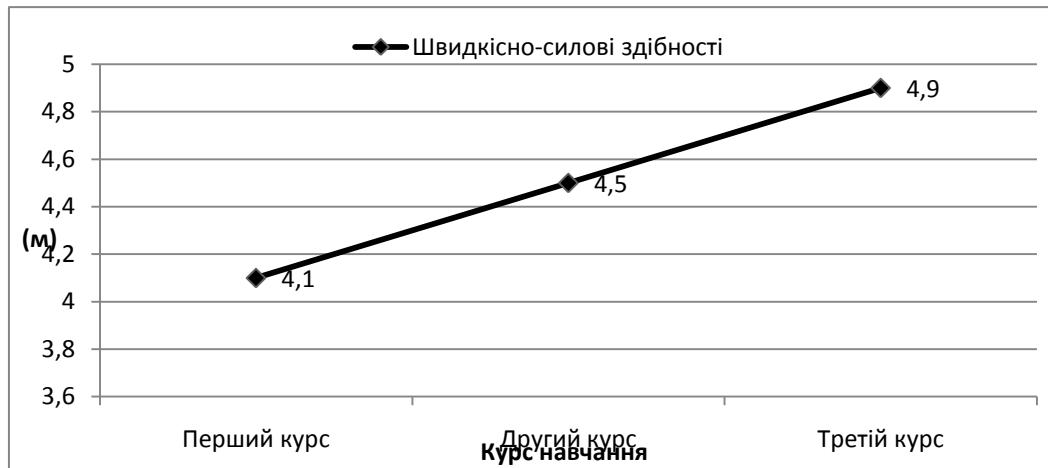
Рис. 2 Динаміка показників швидкісно-силових здібностей студенток спеціальної медичної групи упродовж навчання ( n=80 ; m )
