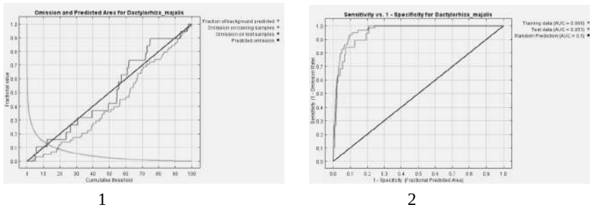
Рис.2. Зміни омісії і передбаченої території моделі за тестовими і тренувальними точкам в залежності від кумулятивного порогу (1) та чутливість і специфічність моделі ареалу D. majalis (2)
