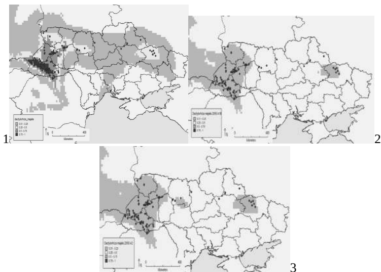
Рис. 3. Моделі потенційних ареалів D. majalis : 1 – сучасний (1975 р.), 2 – 2050 р. (сценарій A1B), 3 – 2050 р. (сценарій A2)
