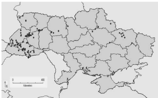
Рис. 1. Локалітети D. majalis , використані для моделювання
