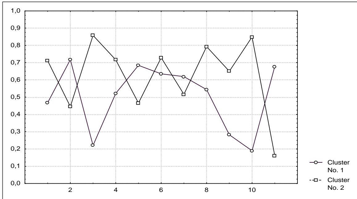
Рис. 2. Кластерний аналіз методом K -середніх.
