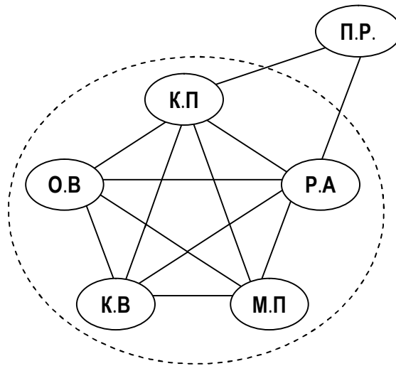
Рис. 8. Асоціативно-ланцюговий кластер
