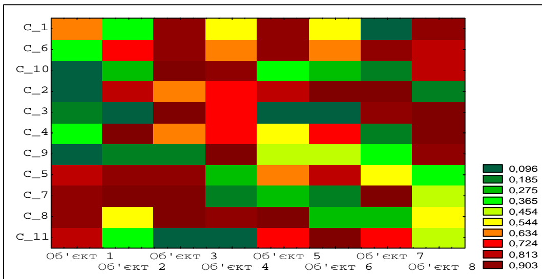
Рис. 3. Результати кластерного аналізу методом двохходового об'єднання
