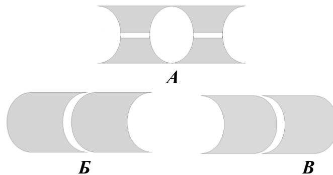
Рис. 48. Хребці амфібій:
