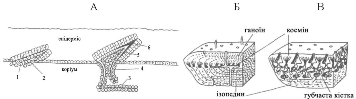
Рис. 20. Типи луски:
