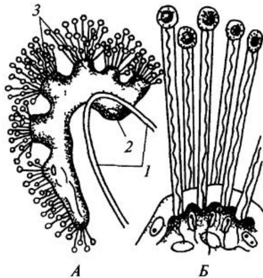
Рис. 6. Нefридії ланцетника:
