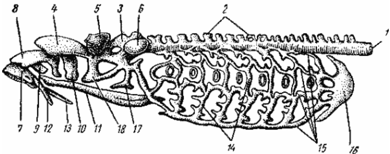
Рис. 15. Скелет міноги:
