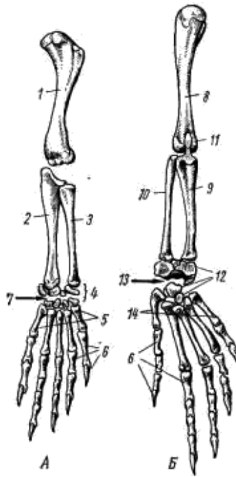
Рис. 75. Кінцівки варана:
