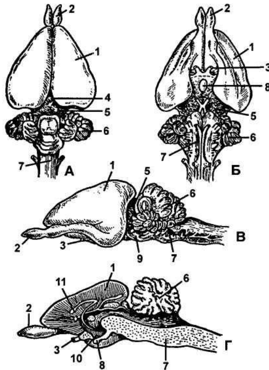
Рис. 118. Мозок кроля:
