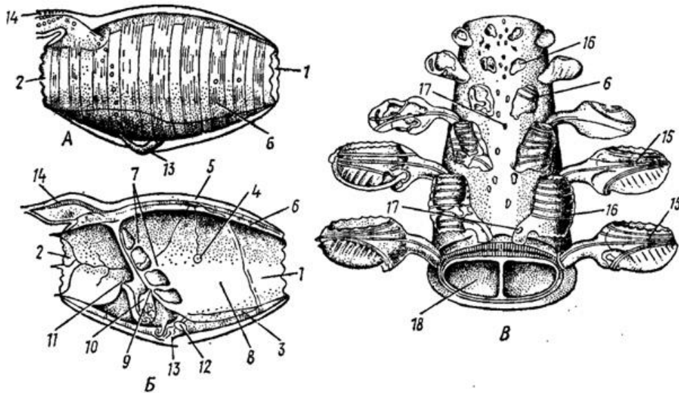
Рис. 9. Сальпи:
