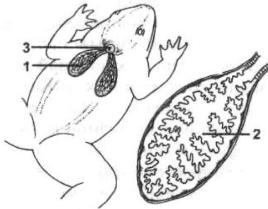
Рис. 55. Легені амфібій:
