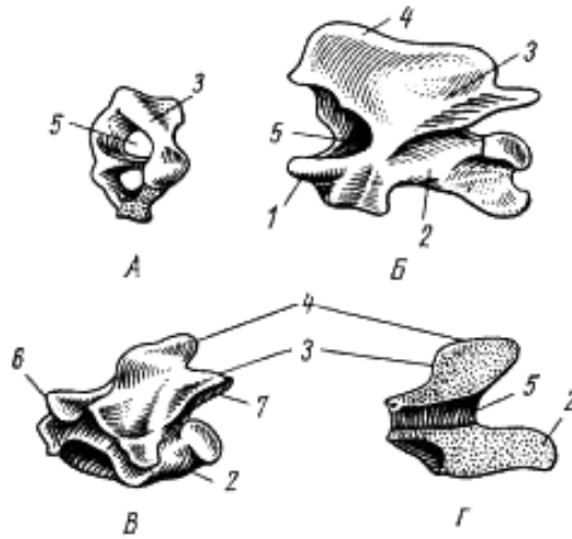
Рис. 70. Хребці варана:
