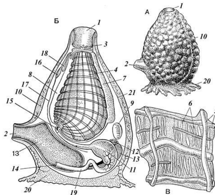
Рис. 7. Будова асцидії:
