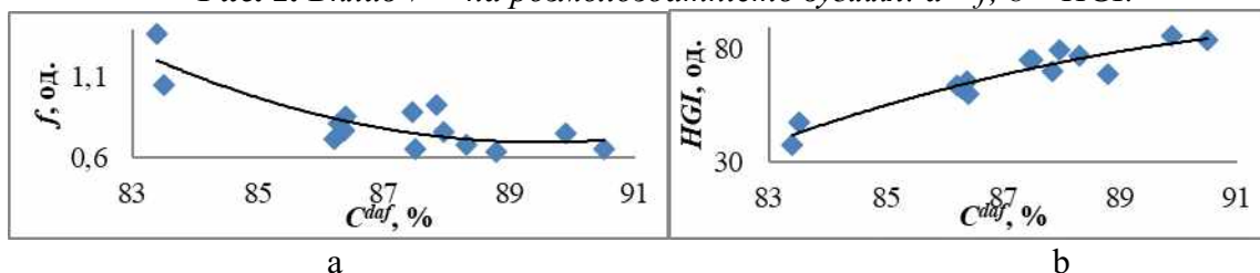
Рис. 3. Вплив C^{daf} на розмолодатність вугілля: а – f ; б – HGI .
