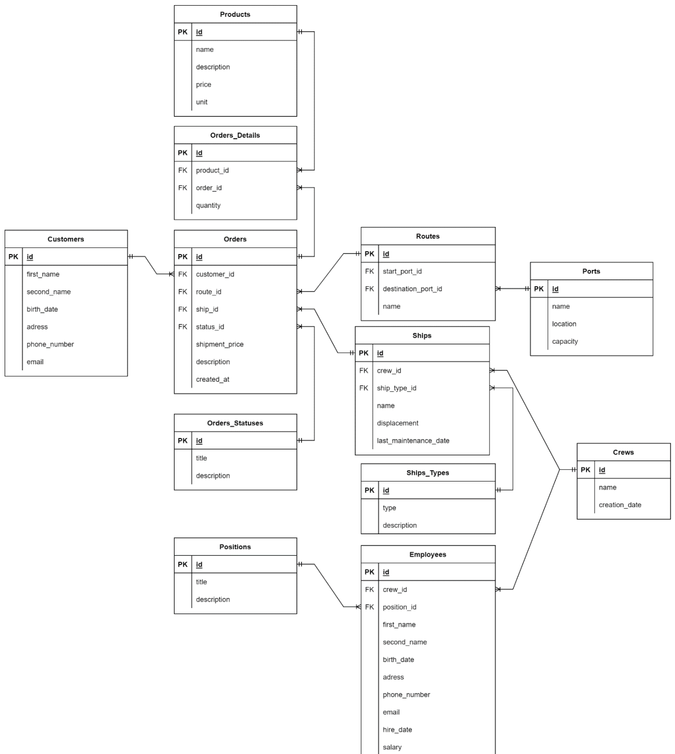
Рис. 1.3 – ER-діаграма
