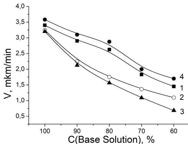
Рис. 4. Залежність швидкості хіміко-механічного полірування CdTe (1), \text{Zn}_{0,04}\text{Cd}_{0,96}\text{Te} (2), \text{Zn}_{0,1}\text{Cd}_{0,9}\text{Te} (3) та \text{Cd}_{0,2}\text{Hg}_{0,8}\text{Te} (4) від розведення базового розчину [в об. %: 12 % \text{HNO}_3 + 88 % KI (ДМФА)] лактатною кислотою.
