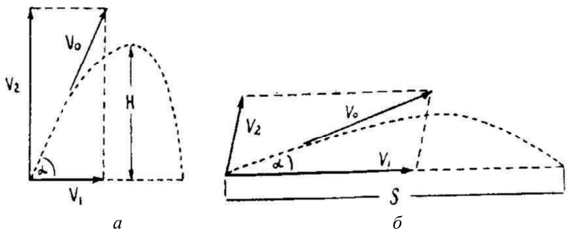
Рис. 2.4. Траєкторія польоту ЗЦМТ:
