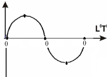
Рис. 2. Ілюстрація нулів функції
