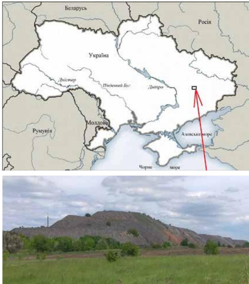
Рис. 1. Картохема району досліджень: проммайданчик із породними відвалами шахти ім. М.І. Сташкова (Петропавлівський район Дніпропетровської області)
