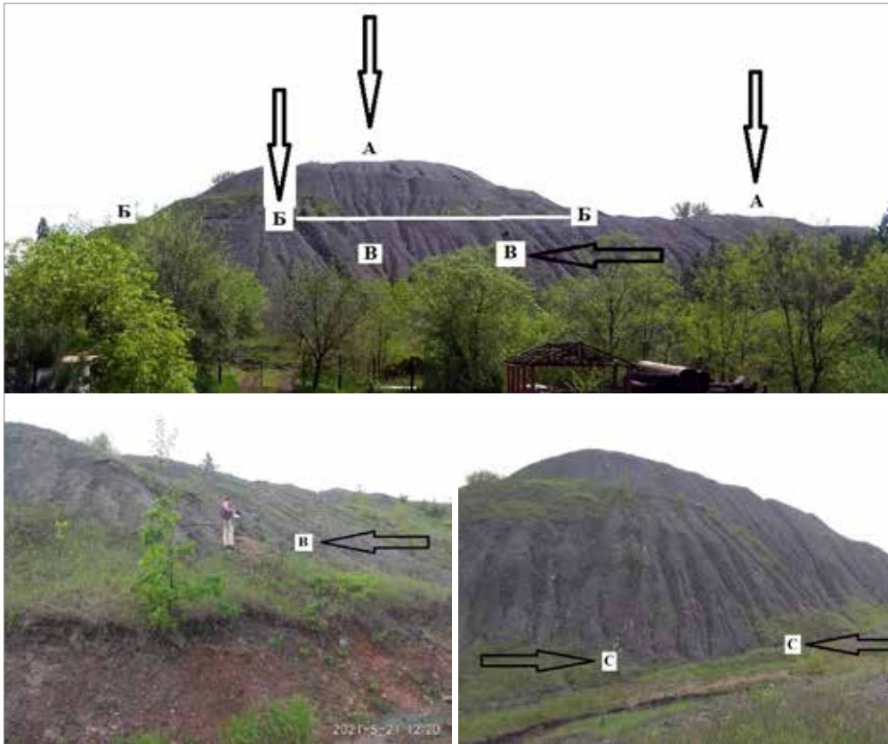
Рис. 3. Складові частини проммайданчика 1, 2, що досліджували: А – плато; Б – тераса; В – схил; С – підосва
