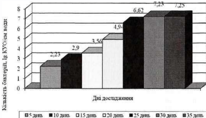
Рис. 15. Кількісні зміни денітрифікуючих мікроорганізмів у воді реактора біофільтра з поліпропіленовим наповнювачем KALDNER KIP за введення його в експлуатацію
