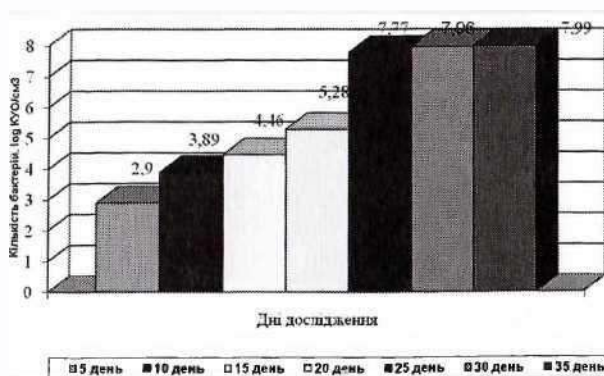
Рис. 8. Кількісні зміни нітрифікуючих мікроорганізмів у воді реактора біофільтра з наповнювачем RK PLAST, за введення його в експлуатацію
