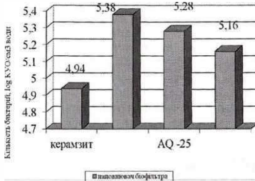
Рис. 11. Середня кількість нітрифікуючих мікроорганізмів у воді реактора біофільтра з різними видами наповнювача за тривалості досліді 30 днів
