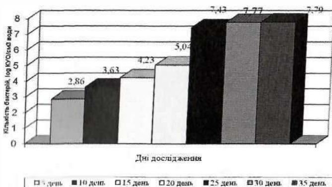
Рис 10. Кількісні зміни нітрифікуючих мікроорганізмів у воді реактора біофільтра з наповнювачем KALDNER K1П, за введення його в експлуатацію
