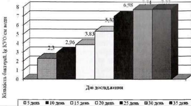
Рис. 13. Кількісні зміни денітрифікуючих мікроорганізмів у воді реактора біофільтра з поліпропіленовим наповнювачем RK PLAST, за введення його в експлуатацію
