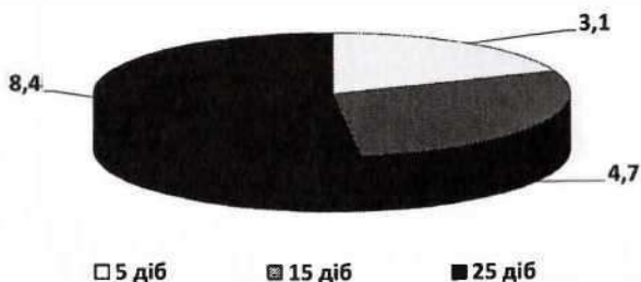
Рис. 3. Динаміка кількості нітрифікуючих мікроорганізмів у воді реактора біофільтра за використання наповнювача Kar-sib (log КУО/см 3 )
