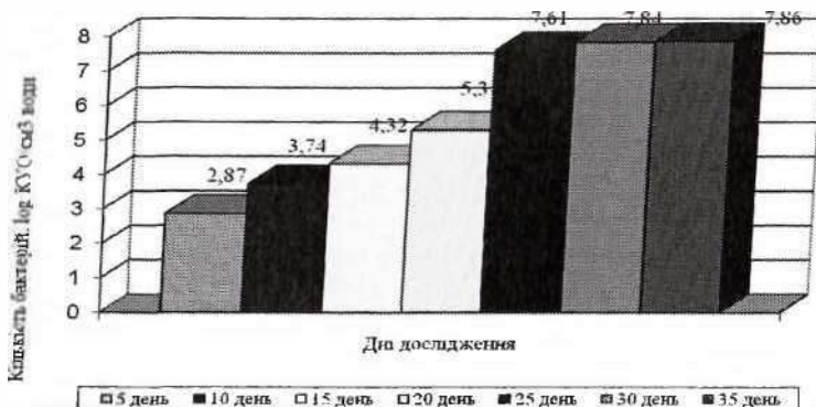
Рис. 9. Кількісні зміни нітрифікуючих мікроорганізмів у воді реактора біофільтра з наповнювачем AQ-25, за введення його в експлуатацію
