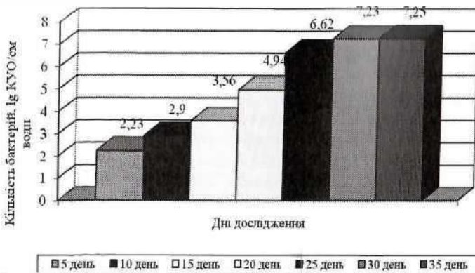
Рис. 12. Кількісні зміни денітрифікуючих мікроорганізмів у воді реактора біофільтра з керамзитовим наповнювачем за введення його в експлуатацію
