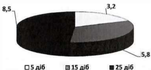
Рис. 2. Динаміка кількості нітрифікуючих мікроорганізмів у воді реактора біофільтра за використання наповнювача АQ-15 (log КУО/см 3 )
