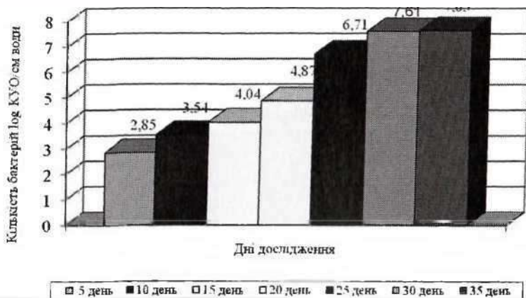
Рис. 7. Кількісні зміни нітрифікуючих мікроорганізмів у воді реактора біофільтра з керамзитовим наповнювачем за введення його в експлуатацію
