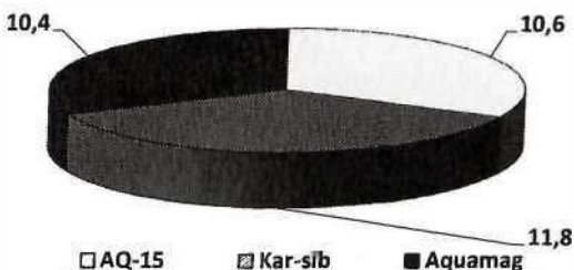
Рис. 5 Зміни кількості нітрифікуючих мікроорганізмів у воді реактора біофільтра за використання наповнювачів AQ-15, Kar-sib, Aquamag ( \text{lg КУО/см}^3 )
