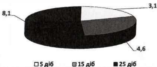
Рис. 4. Динаміка кількості нітрифікуючих мікроорганізмів у воді реактора біофільтра за використання наповнювача Aquamag ( \text{lg КУО/см}^3 )
