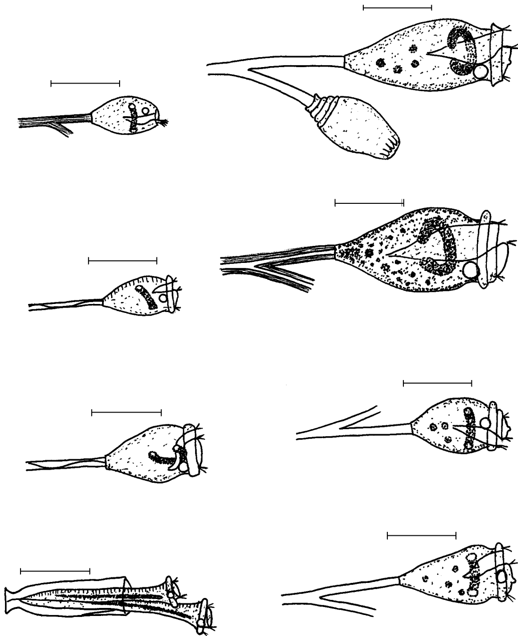
Рис. 1. Перитрихи из аэротенков г. Житомира: 1 — Epistylis coronata ; 2 — E. chrysemydis ; 3 — E. bimarginata ; 4 — E. thinemanni ; 5 — Opercularia microdiscum ; 6 — Vorticella submicrostoma ; 7 — V. peterhoffi ; 8 — Thuricola similis . Масштабна лінійка 50 мкм.
