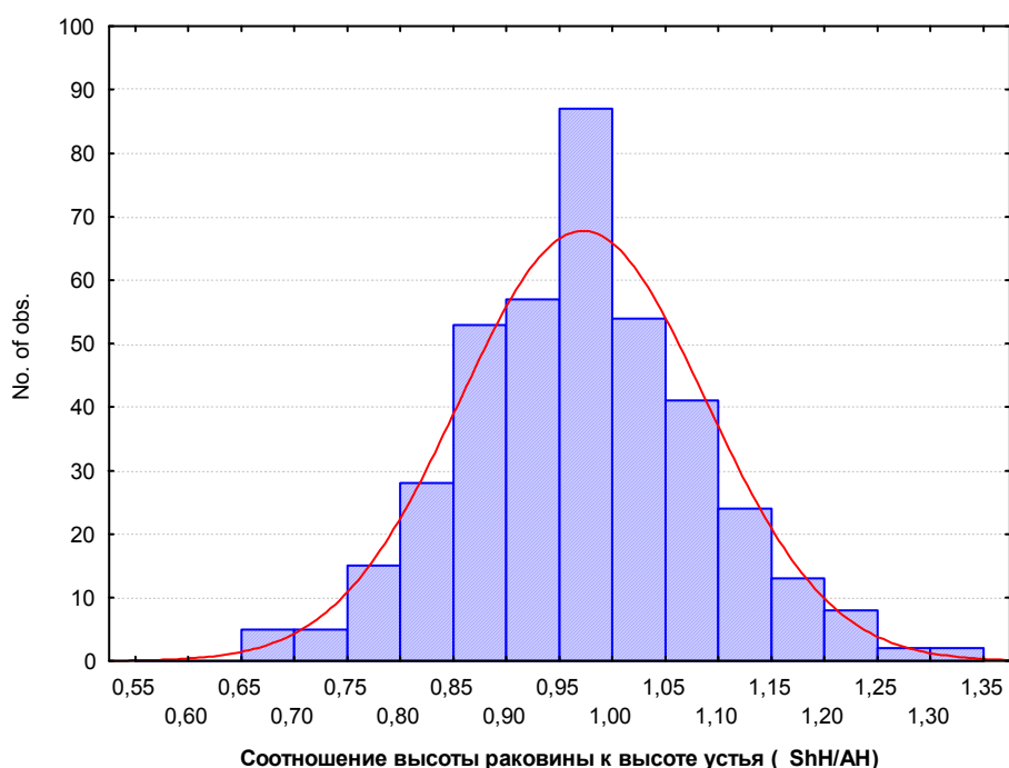
Рис. 4. Распределение значений индекса ShH/АН в обобщенной выборке всех исследованных моллюсков.
