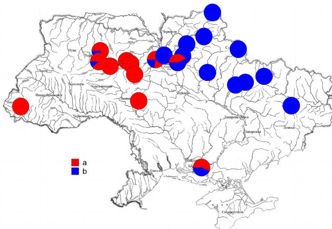
Рис. 3. Распределение аллелей локуса Es-4 по территории Украины.
