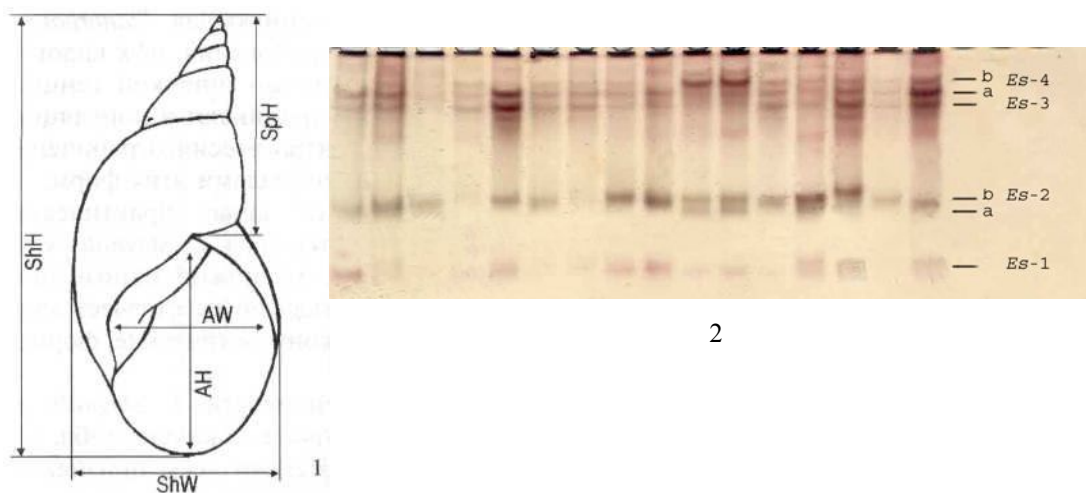
Рис. 1. Схема промеров раковины исследуемых моллюсков: ShH — высота раковины; ShW — ширина раковины; SpH — высота завитка; AH — высота устья; AW — ширина устья.
