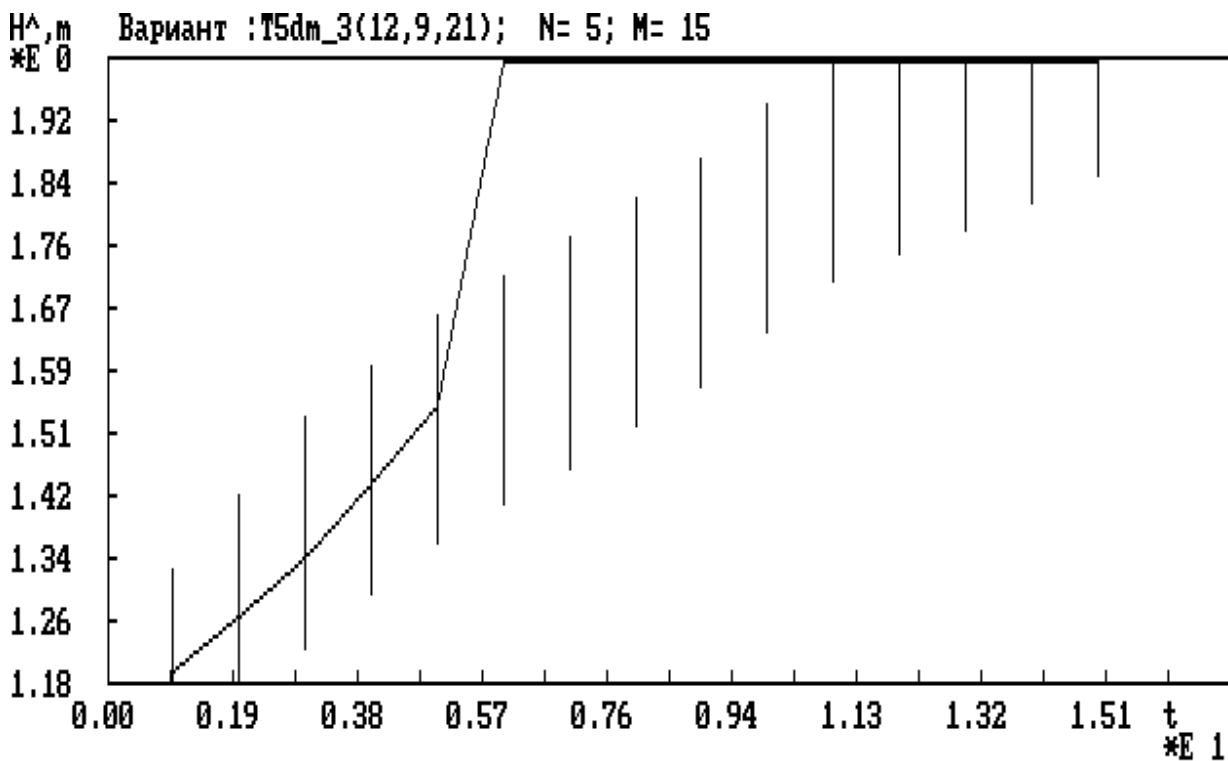
Рис. 4. График регрессии \hat{H}=\hat{H}(t) по трем параметрам ( x_{12} , x_9 , x_{21} ); экспериментальные точки (вертикальные отрезки) поставлены с учетом недопустимо большого среднеквадратичного отклонения CKO=5,1 см (величина отрезков равна 6 CKO ) с интерполяцией параметров на полугодовые периоды
