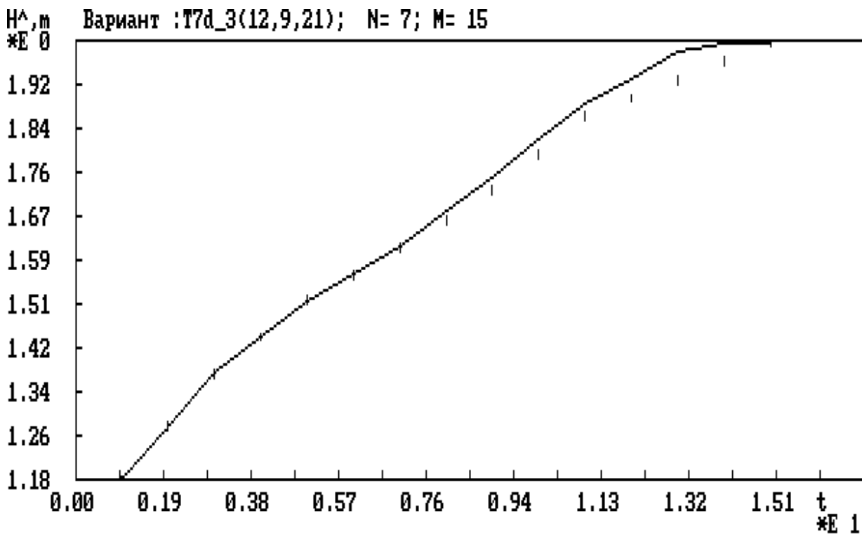
Рис. 2. График регрессии \hat{H}=\hat{H}(t) по трем параметрам ( x_{12} , x_9 , x_{21} ); экспериментальные точки (вертикальные отрезки) поставлены с учетом среднеквадратичного отклонения CKO=0,2\text{см} (величина отрезков равна 6 CKO ) с интерполяцией параметров на полугодовые периоды
