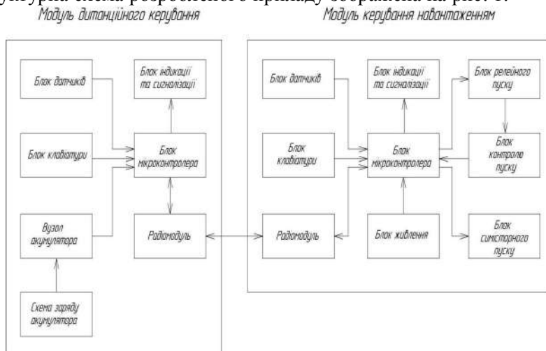
Рис. 1 Структурна схема системи автоматизованого поливу газону
