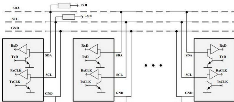
Рис.1 Паралельне підключення пристроїв в шині
