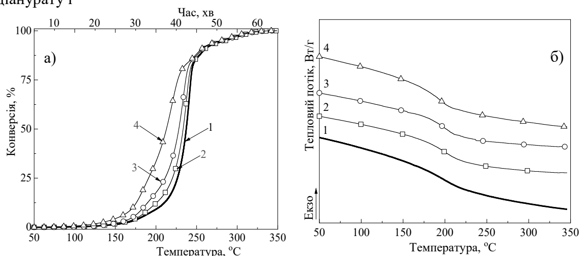
Рис. 3. Температурно-часові залежності конверсії ДЦБЕ/БОА/ЕСН-POSS реакційних сумішей (а) і ДСК термограми ПЦ/ПБА/ЕСН-POSS нанокомпозитів (б), що містять ЕСН-POSS, мас.‰: 1 – 0; 2 – 0,5; 3 – 1,0; 4 – 2,0.
