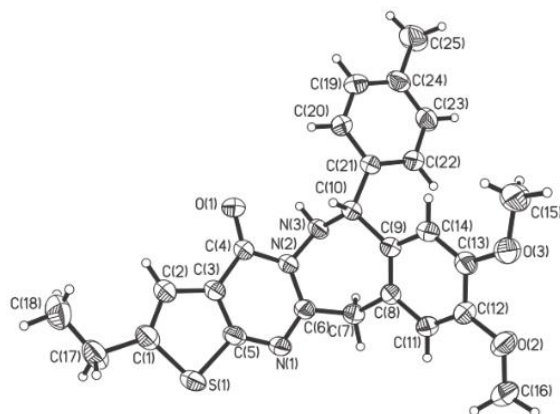
Рис. 1. Структура сполуки 5f за даними РСА.
