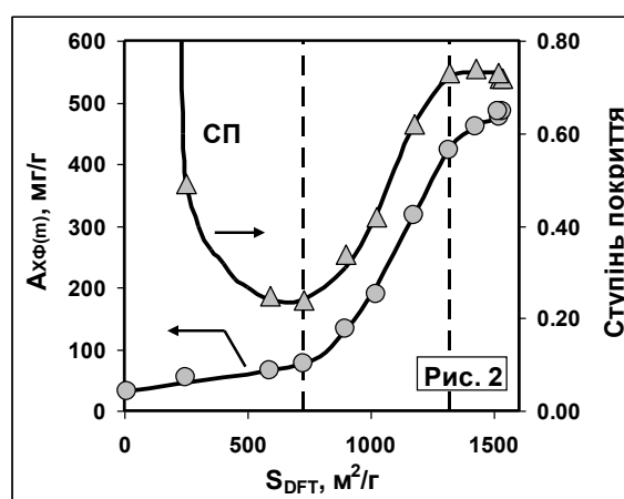
Рис. 2. Залежності максимальної ємності A_{ХФ(m)} та ступеня покриття поверхні від S_{DFT} .
