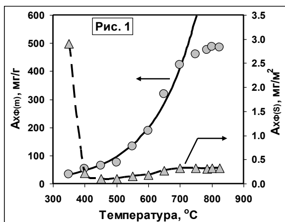
Рис. 1. Ємності A_{ХФ(m)} та A_{ХФ(s)} зразків ВМ, отриманих за різних температур термохемолізу.
