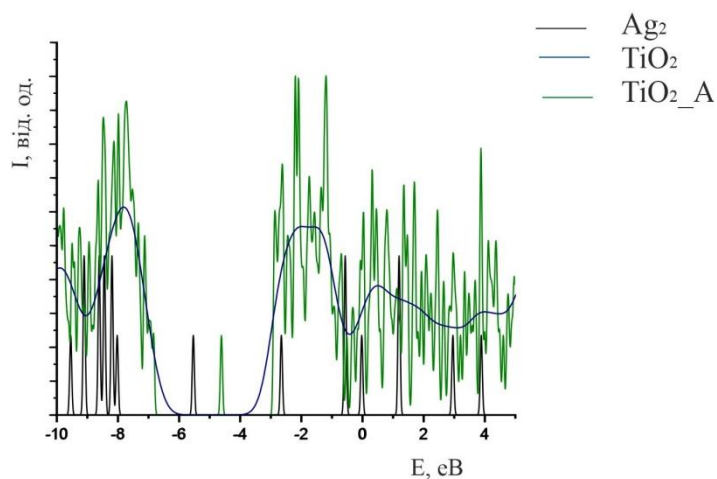
Рис. 2. Спектри одноелектронних станів кластерів \text{Ti}_{15}\text{O}_{41}\text{H}_{22} , \text{Ti}_{15}\text{O}_{41}\text{H}_{22}\text{Ag}_2 та двоатомної молекули \text{Ag}_2
