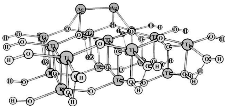
Рис. 1. Рівноважна просторова будова адсорбційного комплексу \text{Ti}_{15}\text{O}_{41}\text{H}_{22}\text{Ag}_2
