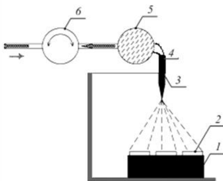
Рис. 1. Схема установки для одержання плівок методом спреї-піролізу.
