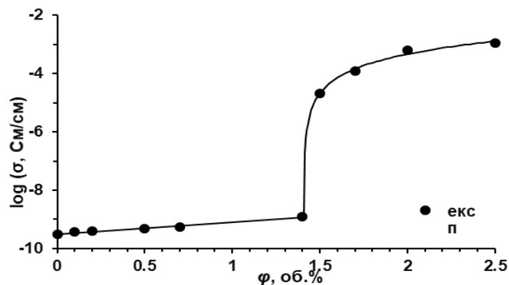
Рис.1. Концентраційна залежності електропровідності композиту ПА-6/БВНТ: експериментальна (точки) та розрахункова (лінія).
