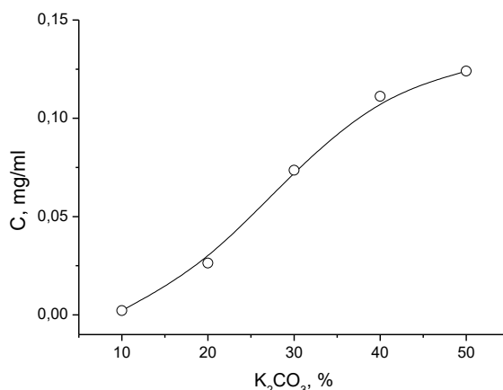
Рис. Залежність концентрації \text{Ti}^{4+} у водному розчині після вилугування при 220^\circ\text{C} протягом 2 годин від відсоткового вмісту \text{K}_2\text{CO}_3 в суміші з \text{KOH} .
