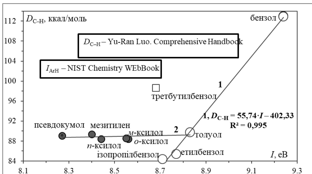
Рис. 1. Залежність між величинами D_{C-H} та I_{ArH} (згідно табл.1) для бензолу і алкілбензолів.
