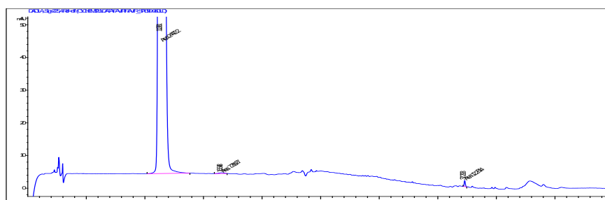
Рис. 3. Хроматограма випробовуваного розчину.
