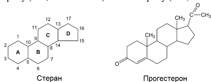
Рис. 1. Хімічні структури стерану і прогестерону.
