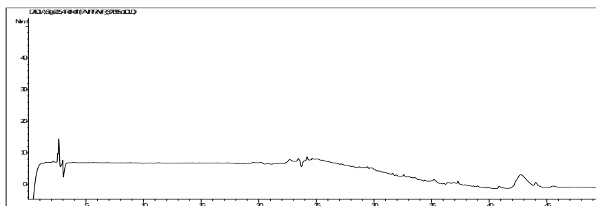
Рис. 1. Хроматограма розчину плацебо.
