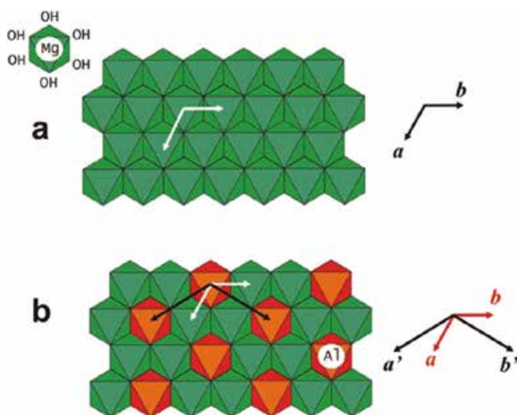
Рис. 1. Буситоподібна структура \text{Mg}(\text{OH})_2
