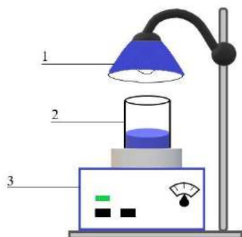
Рис. 1. Установка для проведення фотодеструкції барвників [10]
